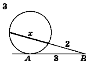
AB — касательная
