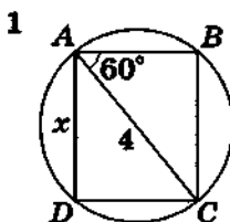
ABCD — прямоугольник
